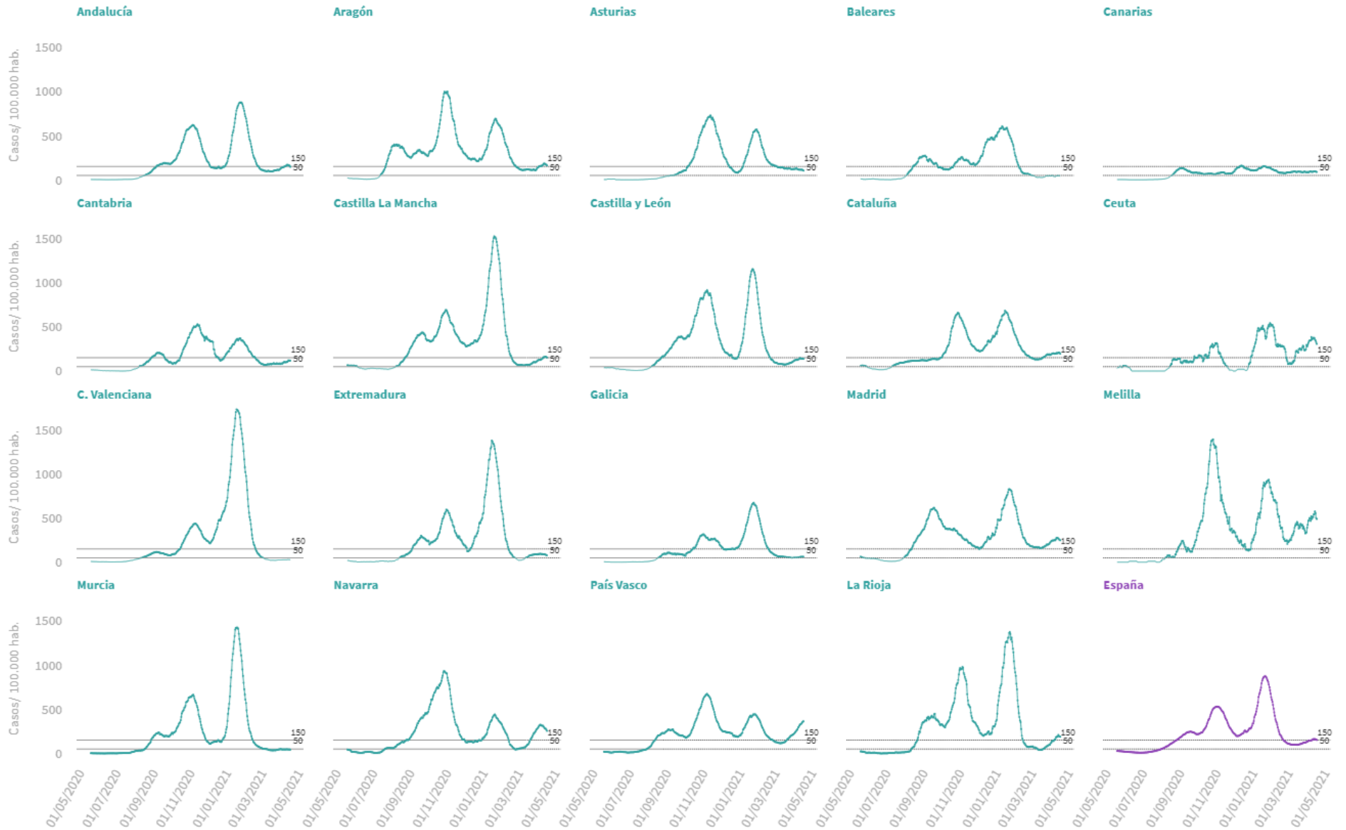
Figura 6. Incidencia acumulada en 14 días en mayores de 64 años por fecha de diagnóstico desde el 11.05.2020 por Comunidades Autónomas, a 22.04.2021 (datos consolidados a las 14:00 horas del 23.04.2021).
